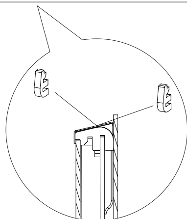
Verwijderen van de binnenruit
