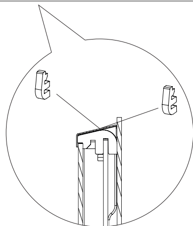
Démontage de la vitre intérieure
