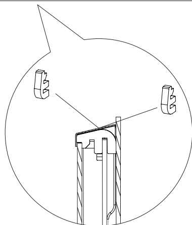
Herausnahme der inneren Scheibe
