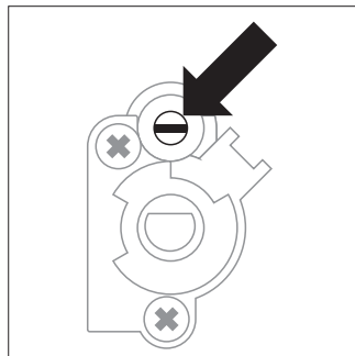
Regulacja zaworu
