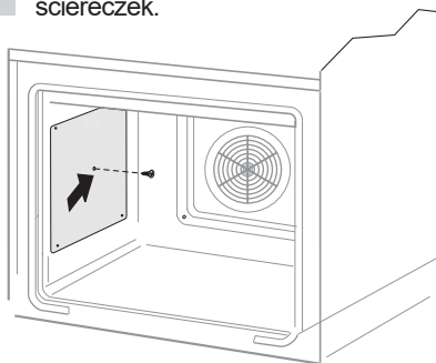
Demontaż wkładek
