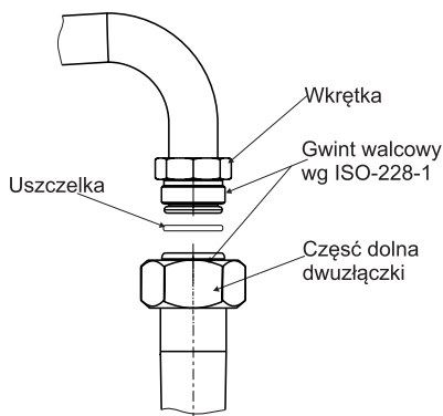
B. Podłączenie za pomocą dwuzłączki.
