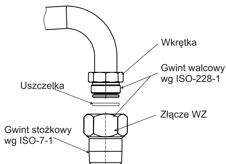
B. Podłączenie za pomocą dwuzłączki.
