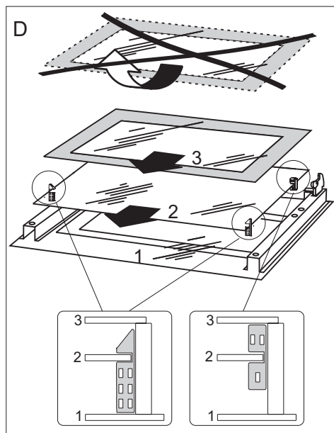
Wyjmowanie szyb wewnętrznych
