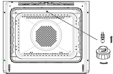
Uunin valaistus
