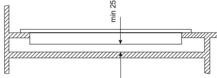
Installation af kogepladen i køkkenbord over skab.
