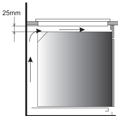
Installation af kogepladen i køkkenbord over ovn med ventilation.
