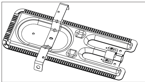
Montáž krytu horáka.
