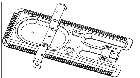
Montáž krytu hořáku.
