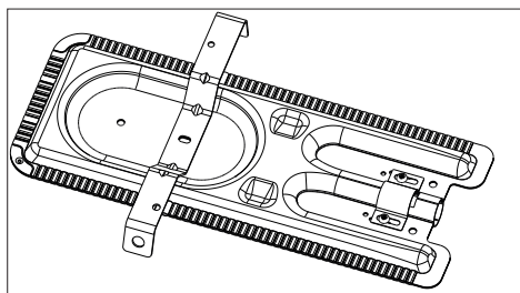
Namestitev zaslonke gorilnika.
