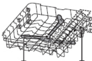
Horní postřikovací rameno
