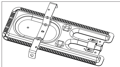
Namestitev zaslonke gorilnika.
