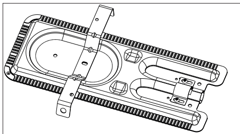
Montáž krytu horáka.
