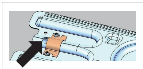
Montaż zasłanki palnika, szczelina 7,5 mm
