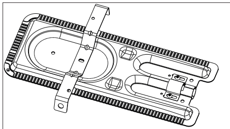
Монтаж на затвора на горелката.
