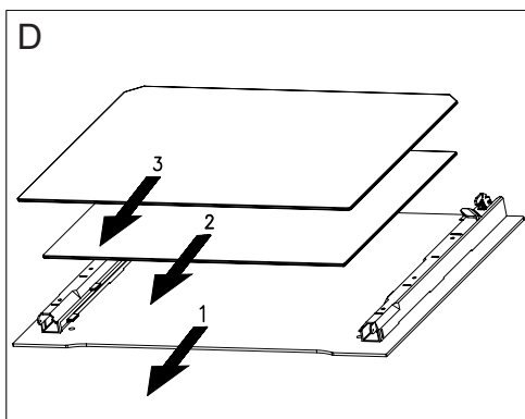
Wyjmowanie szyb wewnętrznych
