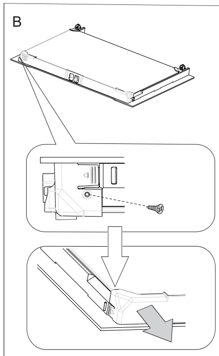
Odchylenie zabezpieczeń zawiasów
