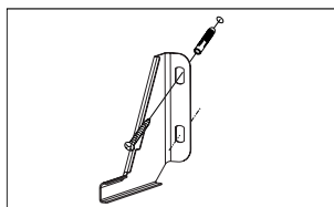
Sporák, výška 900 mm A=123 mm B=166 mm
