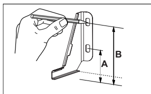
Sporák, Výška 850 mm A=80 mm B=123 mm
