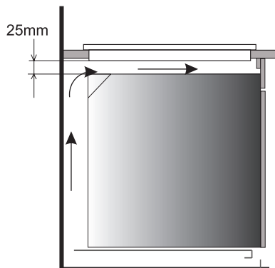
Vgradnja v pult kuhinjske omarice nad pečico
