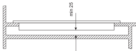
Vgradnja v pult kuhinjske omarice.
