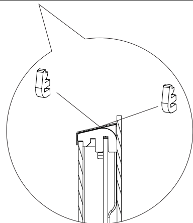
Vyjímání vnitřních skleněných tabulí
