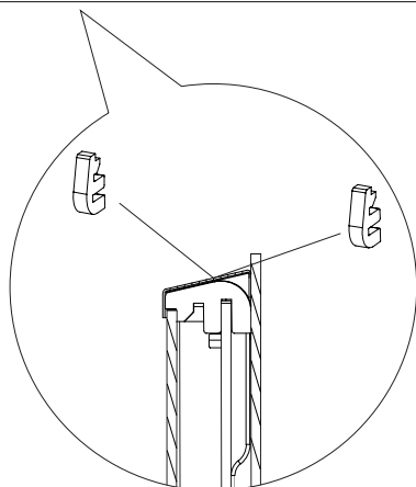
Odstranjevanje notranjih stekel.
